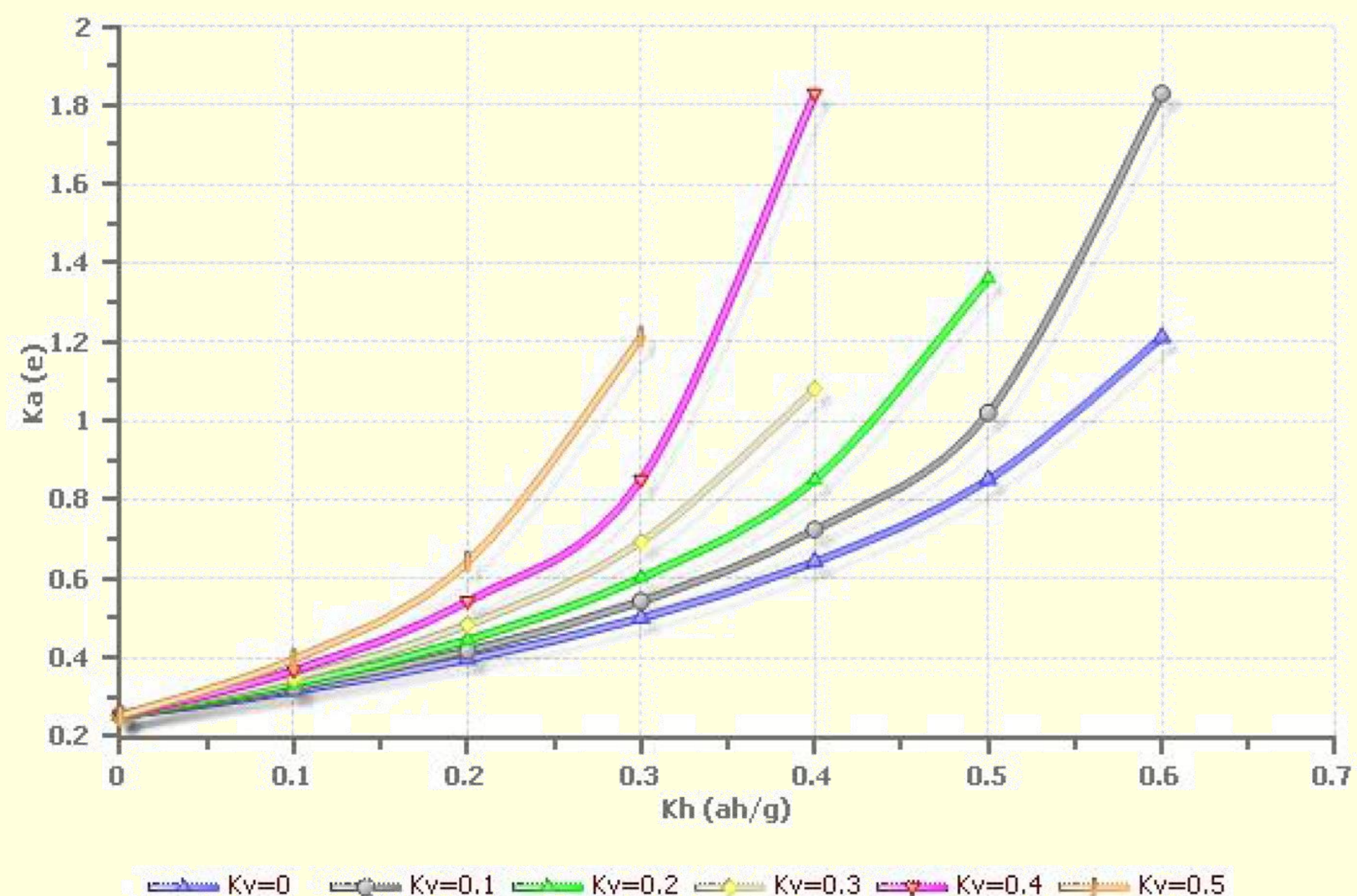
Mononobe-Okabe K_{pa}
